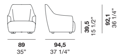
Poltrona con piedini / Armchair with feet
