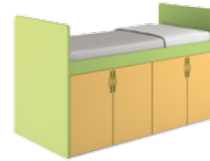
Letto Polar letto con 4 ante battenti DIMENSIONI / SIZES L.2050 P.990 H.1210 mm (rete / bedspring 900x1950)
